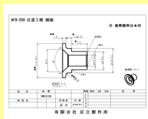
製品図
