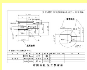
金型図
