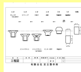
製品工程図
